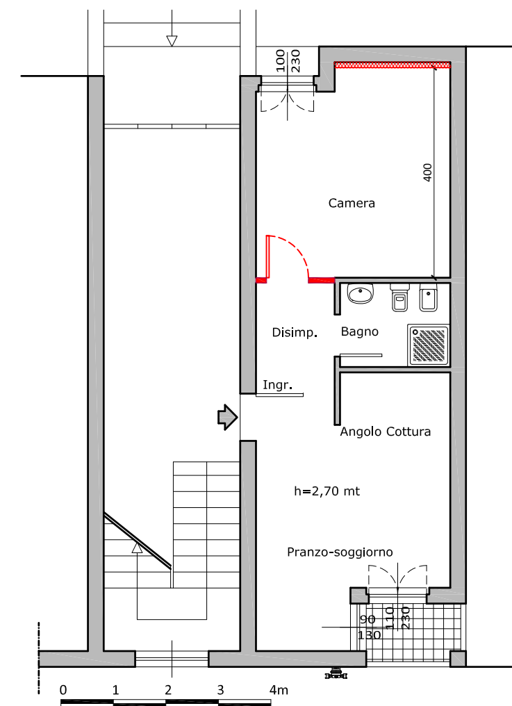
PIANTA PIANO TERRA Sovrapposto tra Stato di fatto e Stato di progetto (Art. 136 comma 6, L.R. 65/2014)
