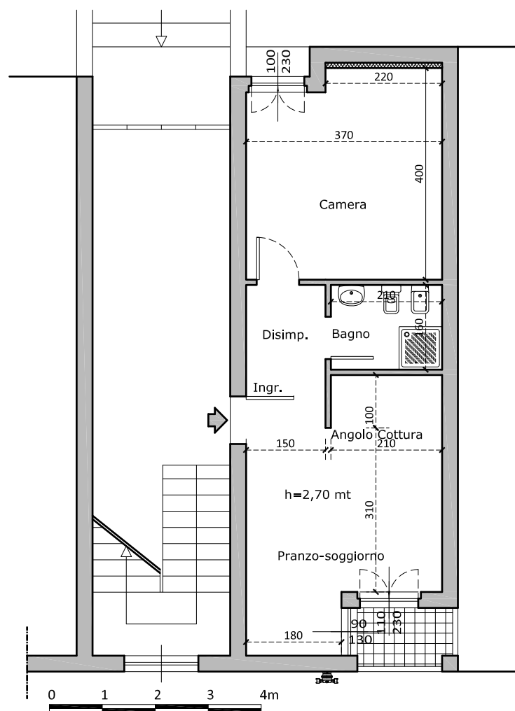
PIANTA PIANO TERRA - STATO DI PROGETTO
