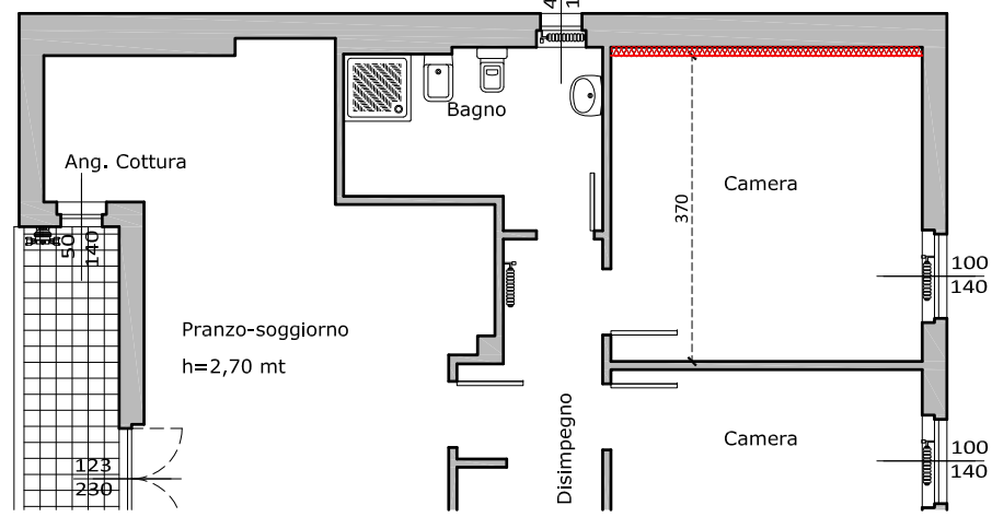
PIANTA PIANO TERRA - Sovrapposto tra Stato di fatto e Stato di progetto (Art. 136 comma 6, L.R. 65/2014)
