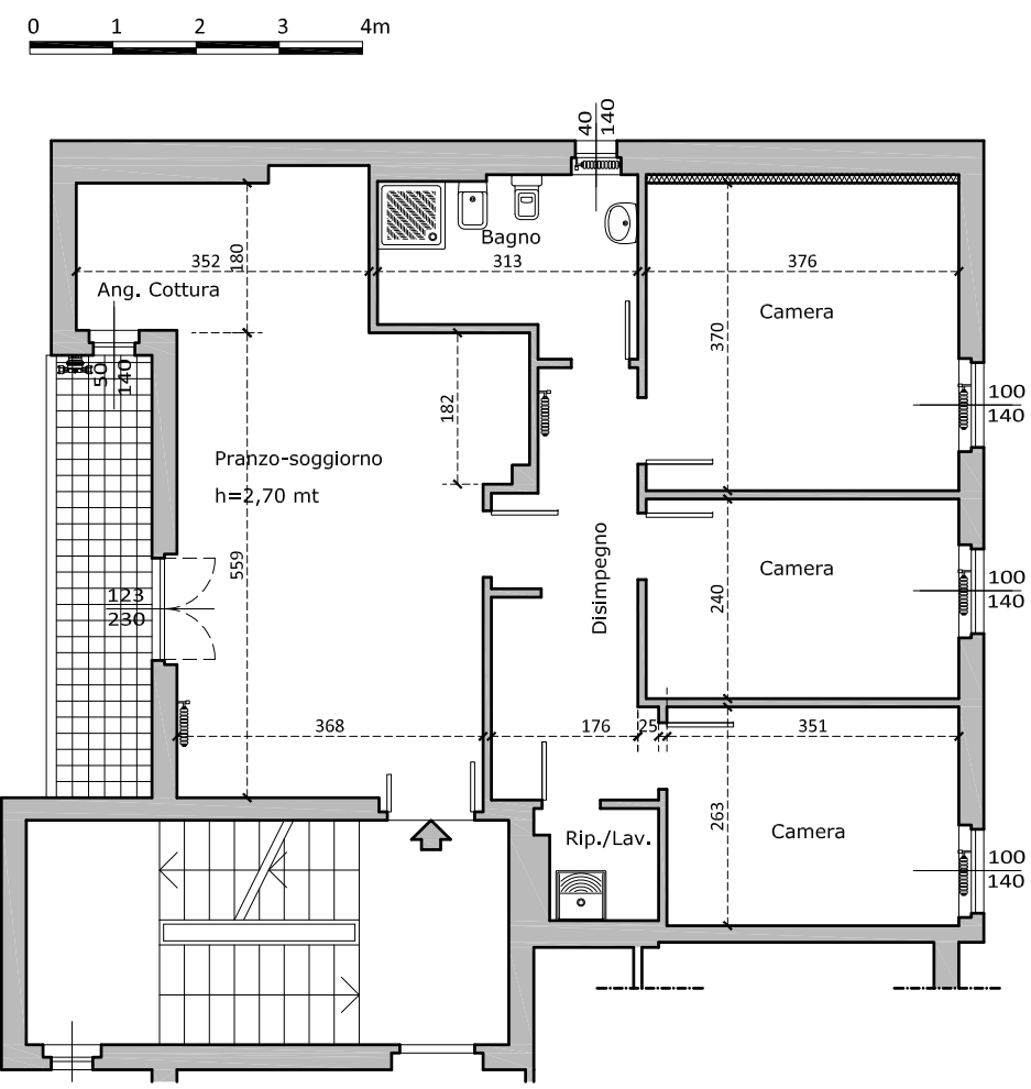
PIANTA PIANO TERRA - STATO DI PROGETTO
