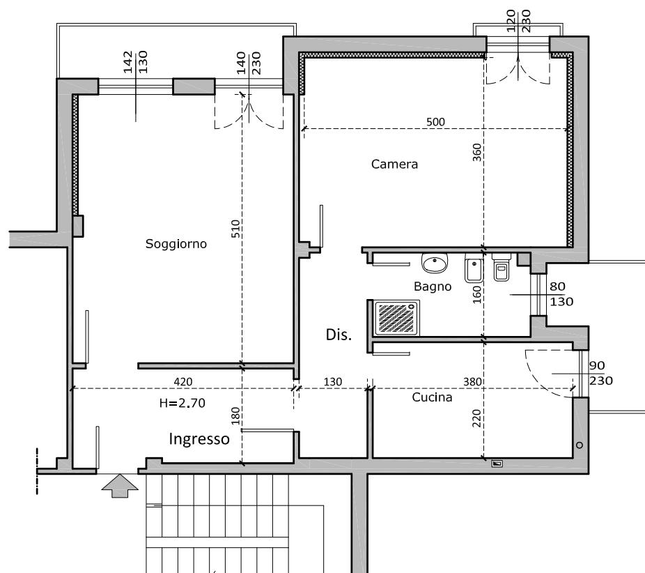
PIANTA PIANO RIALZATO - STATO DI PROGETTO
