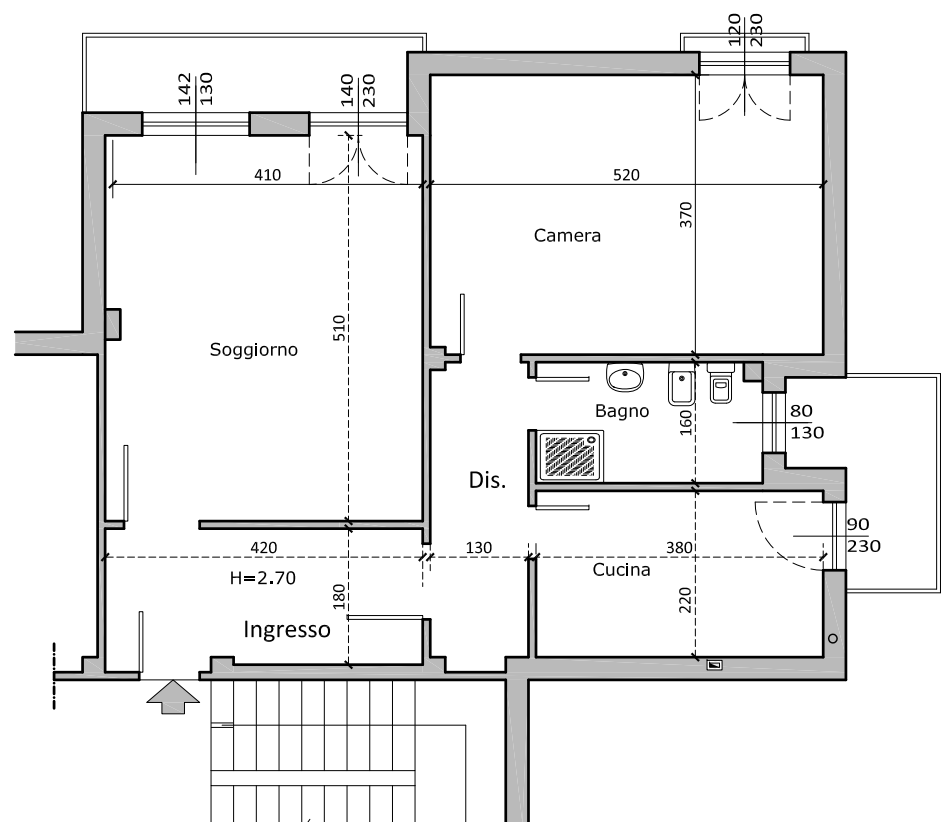
PIANTA PIANO RIALZATO - STATO ATTUALE
