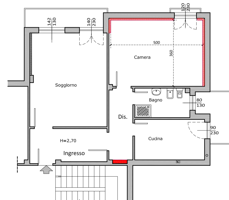
PIANTA PIANO RIALZATO Sovrapposto tra Stato di fatto e Stato di progetto (Art. 136 comma 6, L.R. 65/2014)
