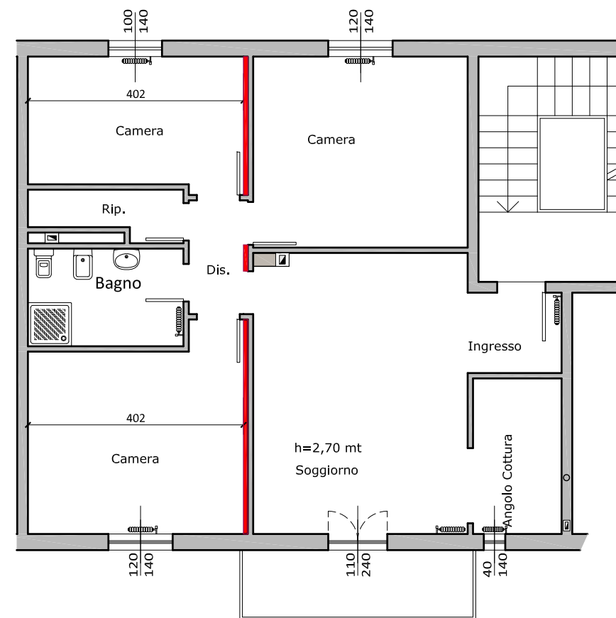
PIANTA PIANO TERZO Sovrapposto tra Stato di fatto e Stato di progetto (Art. 136 comma 6, L.R. 65/2014)
