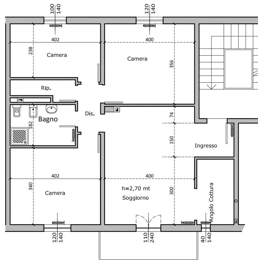
PIANTA PIANO TERZO - STATO DI PROGETTO
